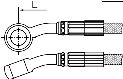
Ringfitting, 20°+20°seitlich lks Alu
