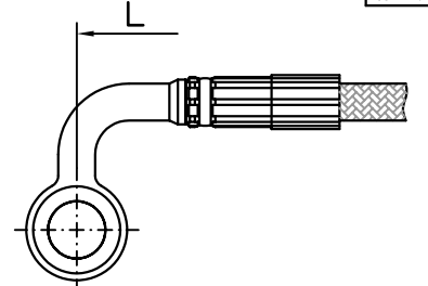
Ringfitting, lang, seitlich 90° Alu
