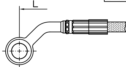
Ringfitting, lang, seitlich 45° Alu
