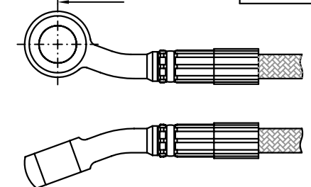
Ringfitting, 20°+20°seitlich rts Alu
