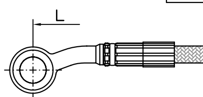
Ringfitting, seitlich 20° Alu
